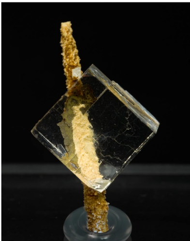
Fluorite - Dalnegorsk, Russia 2.4 x 1.4 cm.
