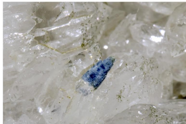
Bazzita - Bonneval, FRANÇA Cristall: 0.2 x 0.1 cm.
