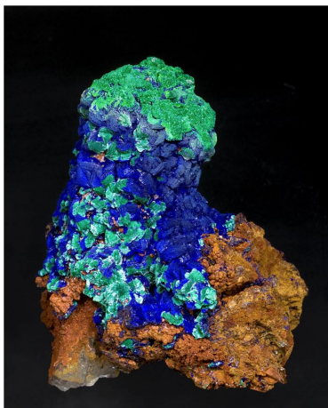
Atzurita - M'Cissi, MARROC 7.2 x 5.9 cm.
